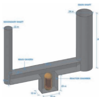
Slika 4. Primer računske analize vplivov potresnih obtežb na stabilnost jaskov majhne podzemne nuklearke [5].
