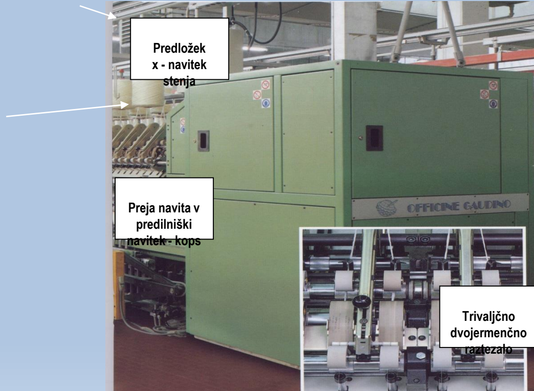
Slika 2.26: Zgradba prstanskega predilnika za izdelavo volnene česanke firme Gaudino
