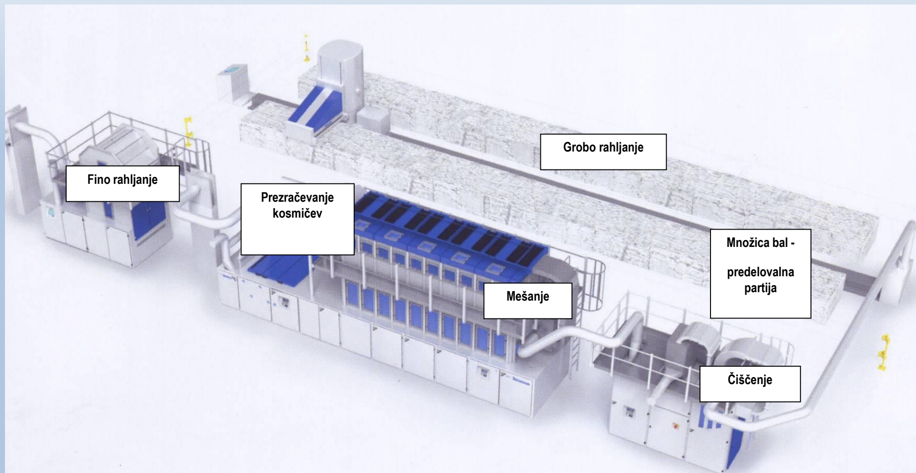
Slika 2.1: Zaporedje strojev za pripravo bombažnega prediva firme Trütschler
