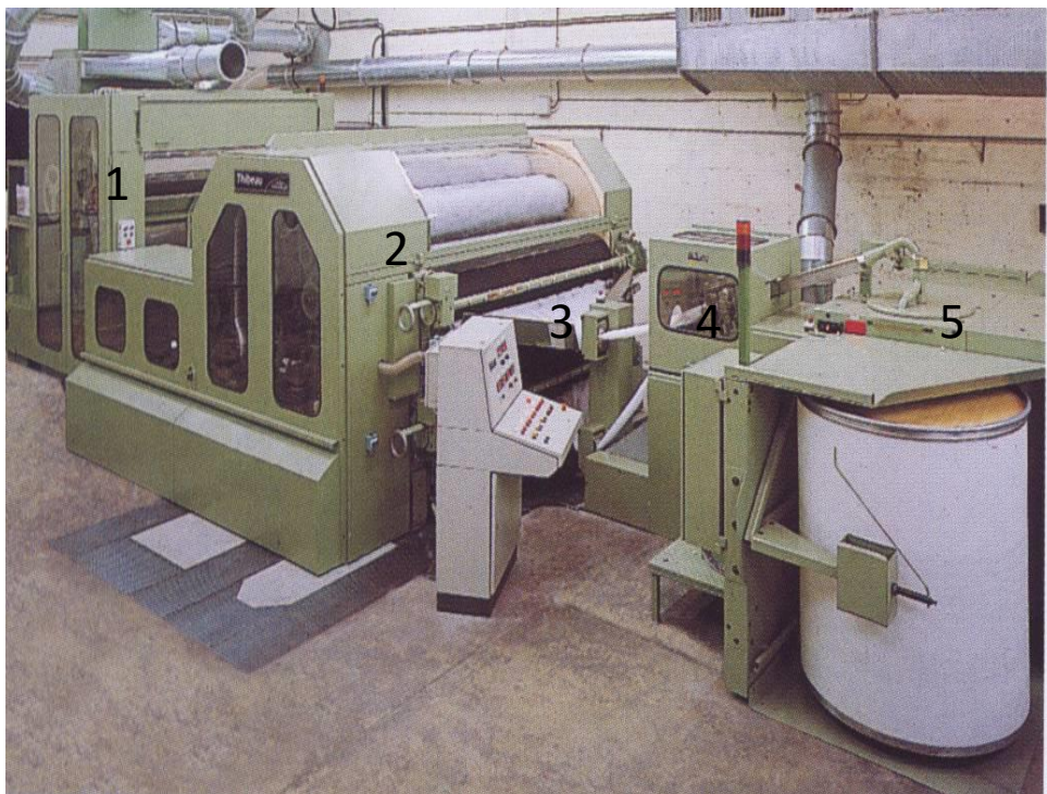
Slika 2.15: Zgradba valjčnega mikalnika za volneno polčesanko firme Schlumberger 1- napajalnik mikalnika 2- valjni mikalnik 3- preoblikovalo koprene v pramen 4- trivaljčno raztezalo pramena 5- odlagalo pramena v lonec
