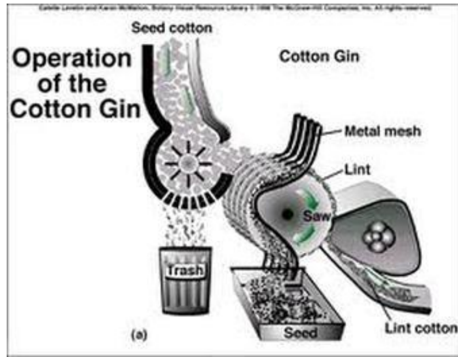
Odzrnjevanje bombaža
