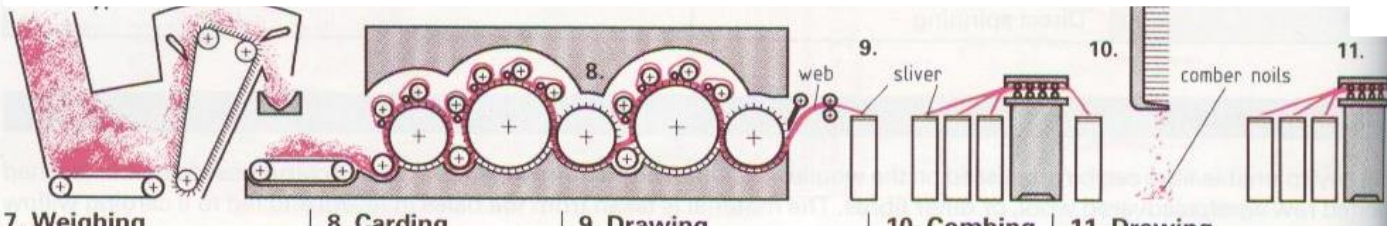
7. Napajalnik mik. 8. Mikanje 9. Raztezanje 10. Česanje 11. Raztezanje po česanju
