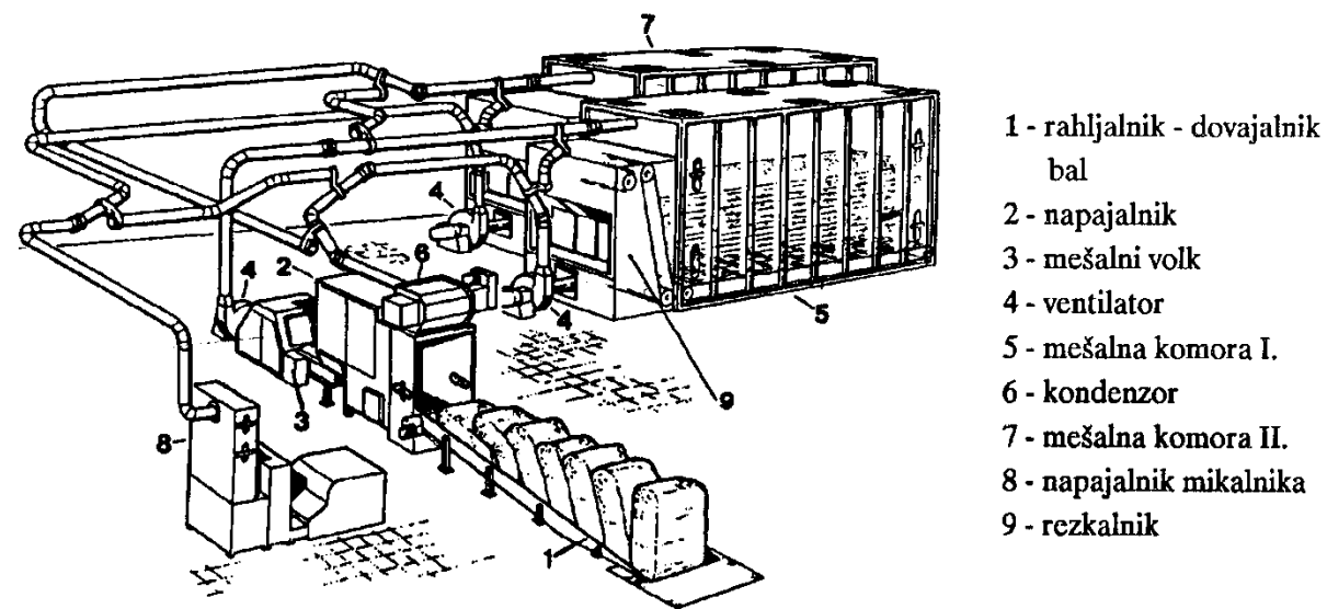
Slika 4.17: Avtomatizirana mešalnica za dolgovlaknato predivo
