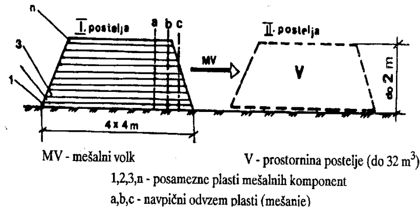
Slika 4.16: Princip mešanja v postelji
