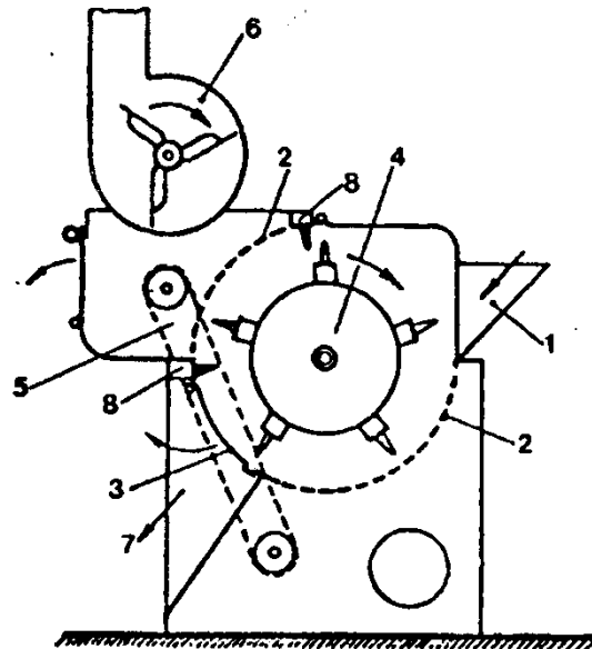
Slika 5.2: Izpraševalnik krp
