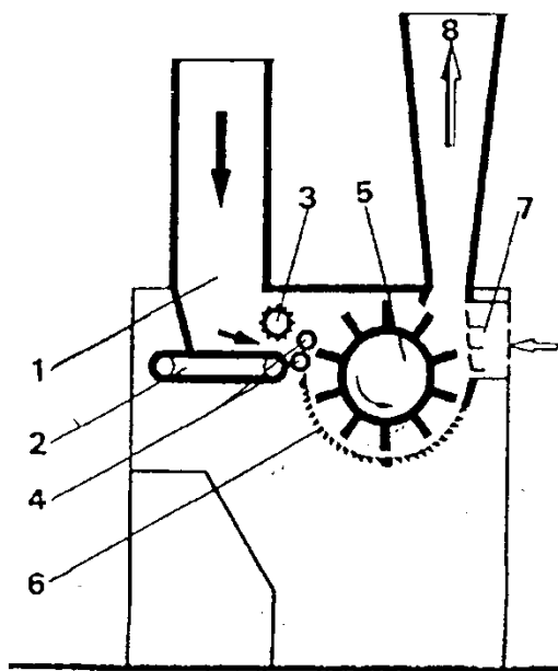
Slika 4.6: Vodoravni rahljalnik z rahljalnimi noži 1- dovod prediva 2- dovajalni transportni trak 3- obtežilni valj 4- dovajalna valja 5- rahljalni boben obložen z noži 6- rešetka 7- dovod zraka 8 pnevmatski transport zrahljanih kosmičev Slika 4.6: Vodoravni rahljalnik z rahljalnimi noži
