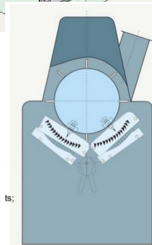
Slika 4.4: Enobobenski aksialni rahljalnik 1- dovod prediva 2- valj z motovili 3- rešetka 4- preusmerjevalna pločevina 5- vijačni tok prediva 6- odvod prediva
