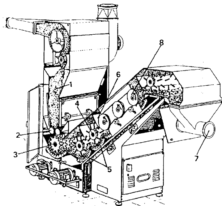
Slika 4.5: Stopenjski rahljalik
