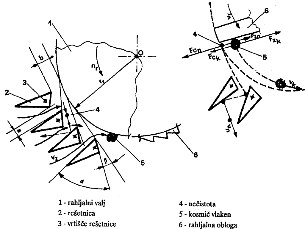
Slika 4.10: Postavitev rešetnic pod rahljalnim valjem in sile, ki delujejo med rahljanjem prediva
