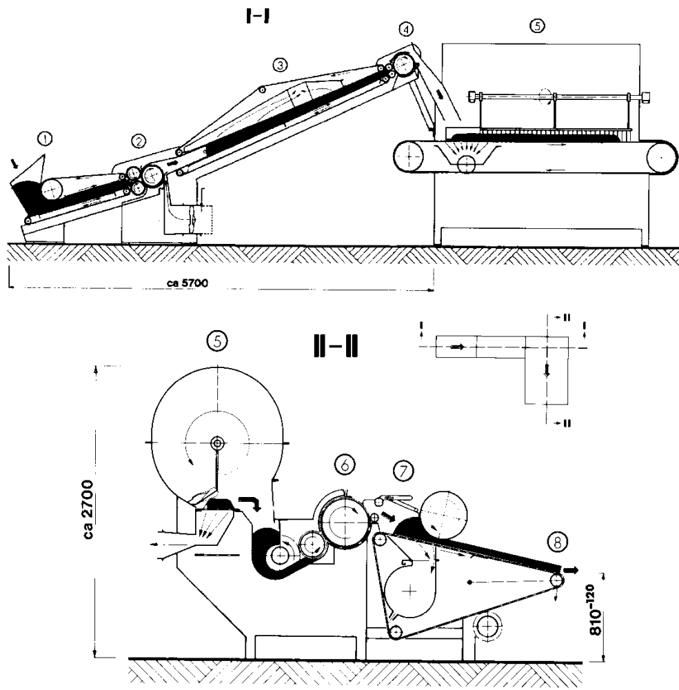
Slika 6.20. Aerodinamični izdelovalnik koprenskega runa V12 firme Fehrer 1- napajalnik 2,4,6- rahljalne enote 3- elevatorski transporter runa 5- razprševalo kosmičev 7- pihalo kosmičev 8- koprensko runo
