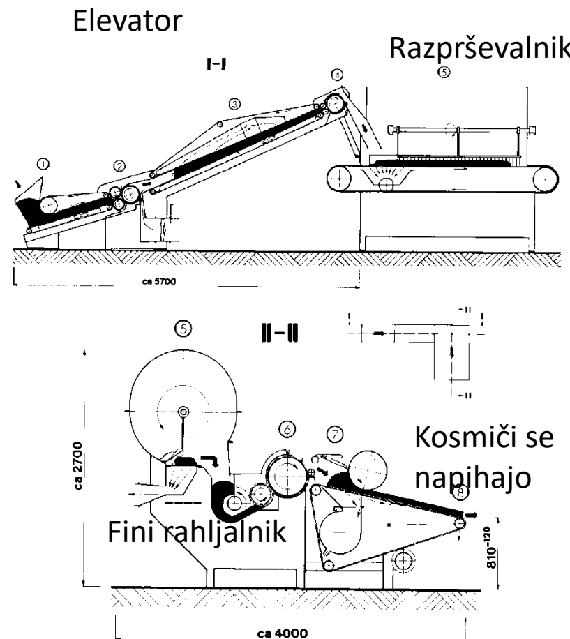
Slika 6.20. Aerodinamični izdelovalnik kopenskega runa V12 firme Fehrer 1- napajalnik 2,4,6- rahljalne enote 3- elevatorski transporter runa 5- razprševalo kosmičev 7- pihalo kosmičev 8- kopensko runo
