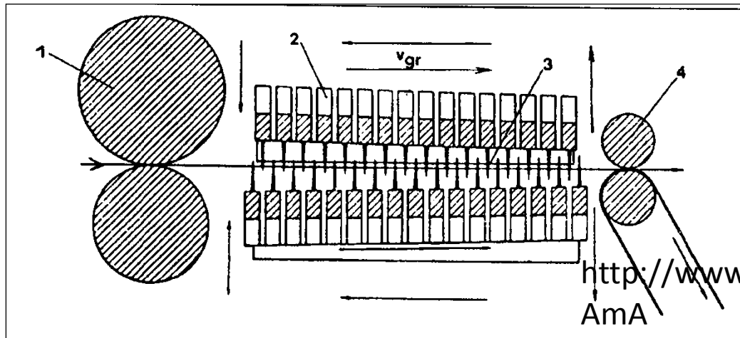
Slika 7.10: Dvopoljsko grebenko raztezalo s potujočimi grebeni
