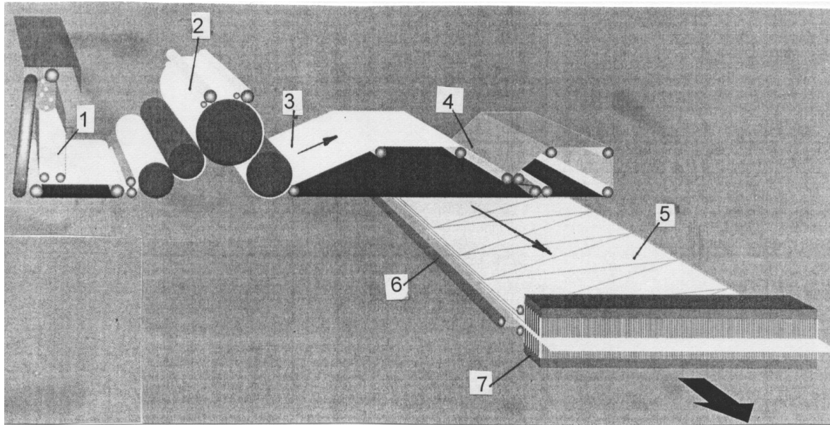
Slika 7.4. Izdelava plastene koprenske tekstilije s križnim polagalnikom (53) 1- napajalnik mikalnika 2- mikalnik 3- transport koprene od mikalnika do polagalnika 4- križni polagalnik 5- plastena koprena ( N_{pl} = 5 do 15 dvojnih plasti) 6- združevalni trak, na katerem se polagajo plasti koprene 7- utrjevalnik, ki mehansko utrdi plasteno kopreno (prediglalnik in/ali iglalnik)
