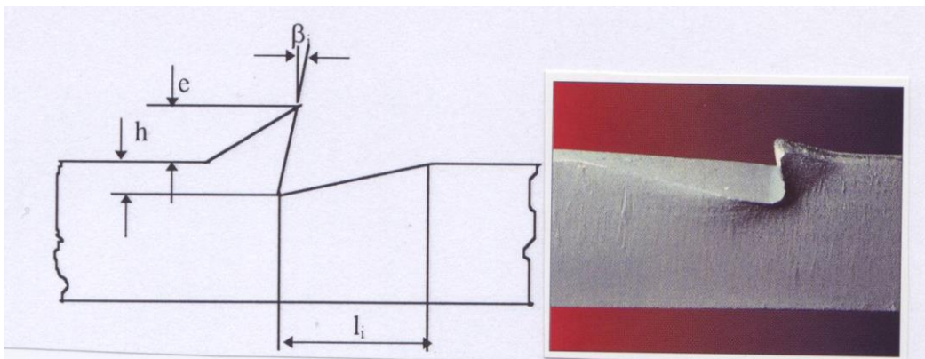
Slika 9.18. Geometrija zazobka (53)
