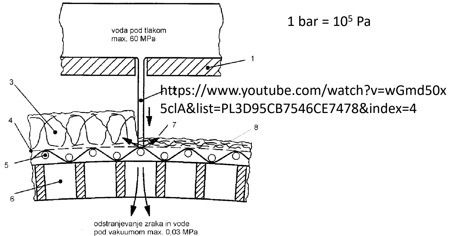
Slika 9.27. Princip utrjevanja z vodnim curkom (53)
