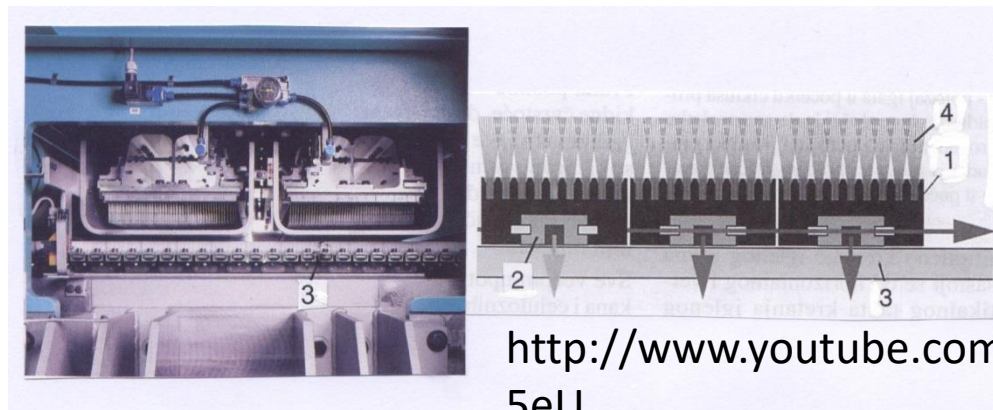
Slika 9.14. Izdelava lasaste strukturirane koprenske tekstilije (53) 1- ščetka 2- magnetno vodilo ščetke 3- brezkončni zobati trak, ki translatorsko premika ščetkasto temeljno desko 4- ščetka iz množice niti iz toge najlonske vrvice (laksa)
