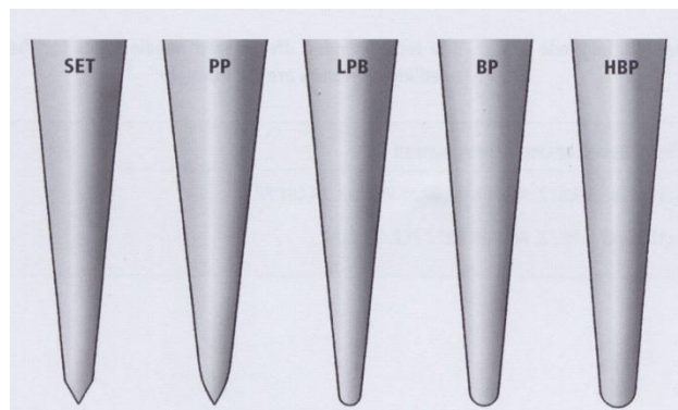
Slika 9.21. Geometrija konice igle firme SNF
