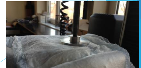
Preskušanje tlačne elastičnosti higienskega izdelka
