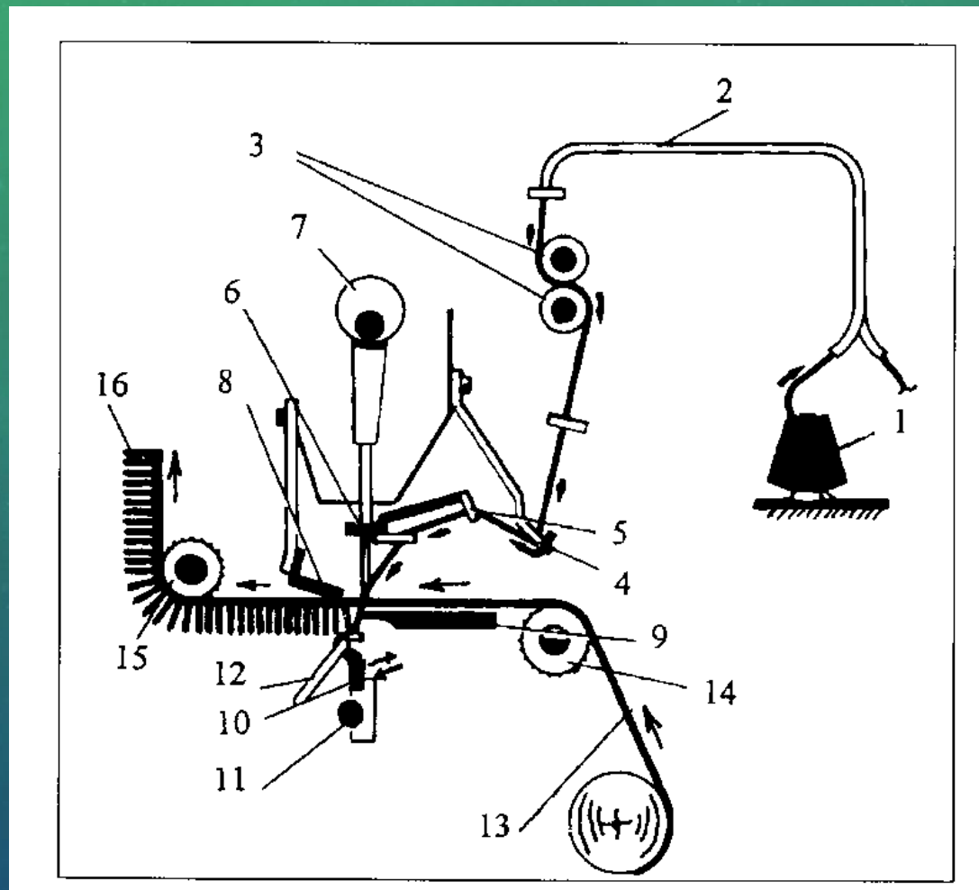
1- navitek preje za tvorbo lica preproge 2- cev za vodenje preje 3- rebrasta dovajalna valjička 4,5- vodilo preje 6- igelna deska z očesnimi iglami 7- ekscentrično gonilo 8- tipalo hrbtne strani taftane preproge 9- luknjana temeljna deska 10- grabilo niti 11- vrtilišče grabila niti 12- nož 13- temeljna tekstilija 14,15- dovajalni, odvajalni valj 16- surova taftana preproga
