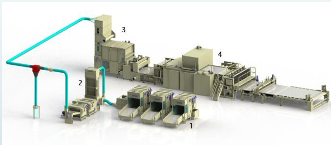
Linija za izdelavo zračno položene netkane tekstilije (Airlay) iz reciklrnih vlaken proizvajalca Laroche, 1 -Rahljalnik bal s poševnim iglastim trakom in tehtalno enoto, 2 – fini vertikalni rahljalnik, 3 Detektor prisotnosti kovin, 4 – Flexiloft airlay sistem
