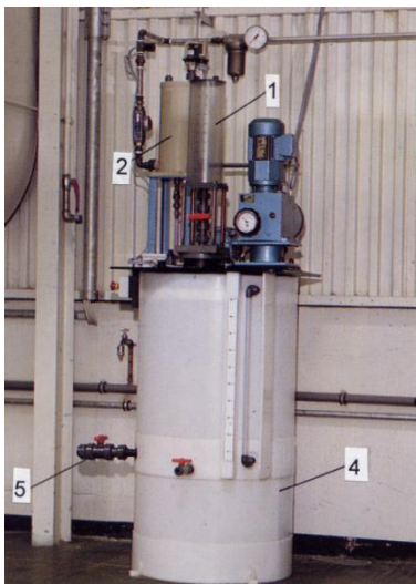
Slika 5.8. Naprava za pripravo mastilne emulzije firme Temafa
