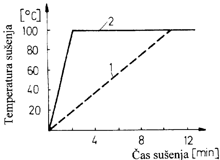
Slika 9.57. Odvisnost temperature ogrevanja od časa
