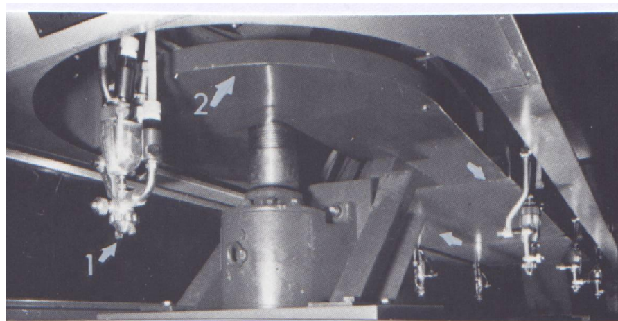
Slika 9.51. Transporter množice brizgalnih šob (53)
