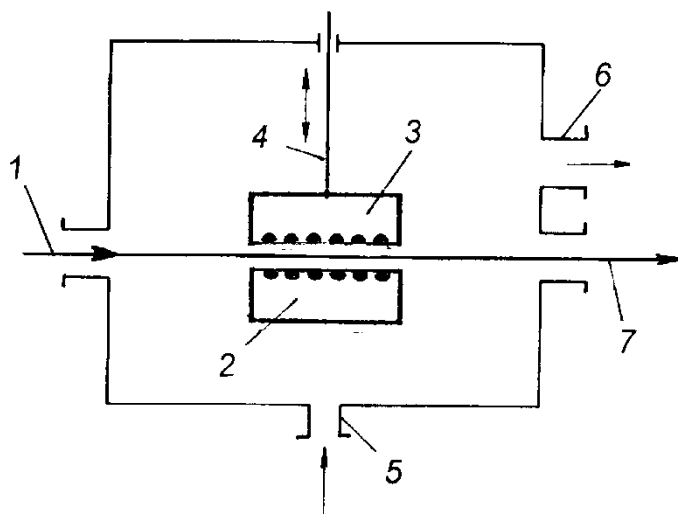
Slika 9.58. Visokofrekvenčni sušilnik
