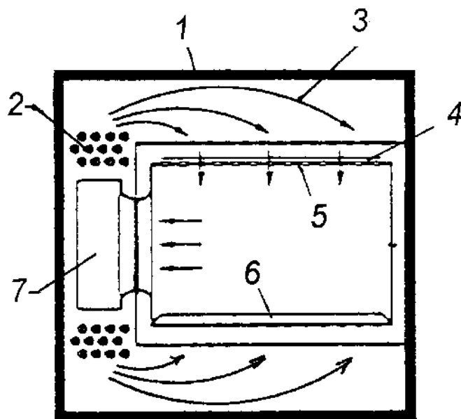
Slika 9.61. Delovna enota sušilnika z luknjanim bobnom firme Fleissner
