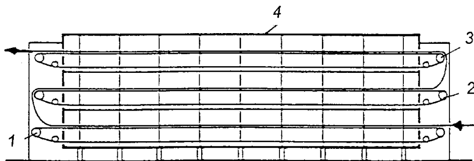
Slika 9.67. Zgradba trietažnega šobnega sušilnika firme Fleissner 1,2,3- prva, druga, tretja etaža sušenja tekstilije
